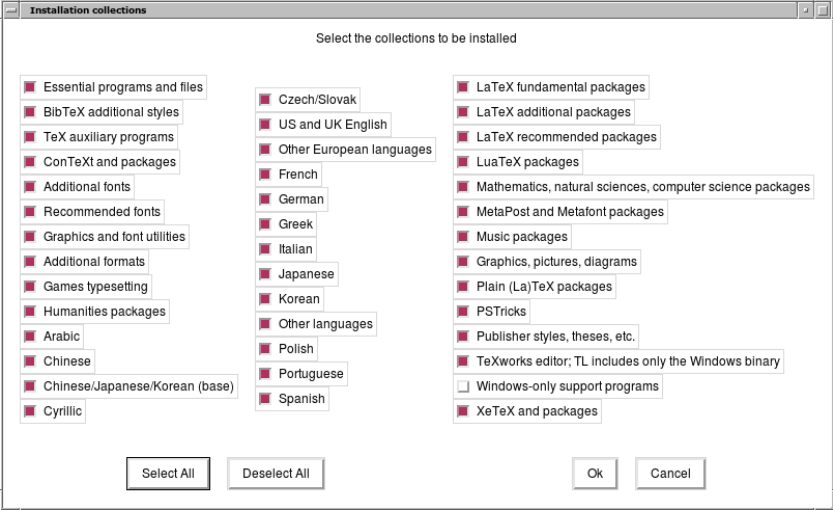
Obrázek 7: Nabídka kolekcí
