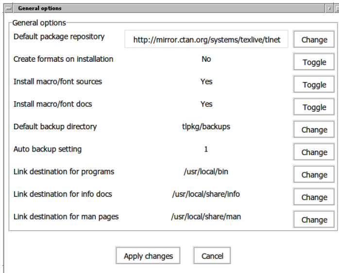
Рис. 10: Программа tlmgr в графическом режиме: главное меню
