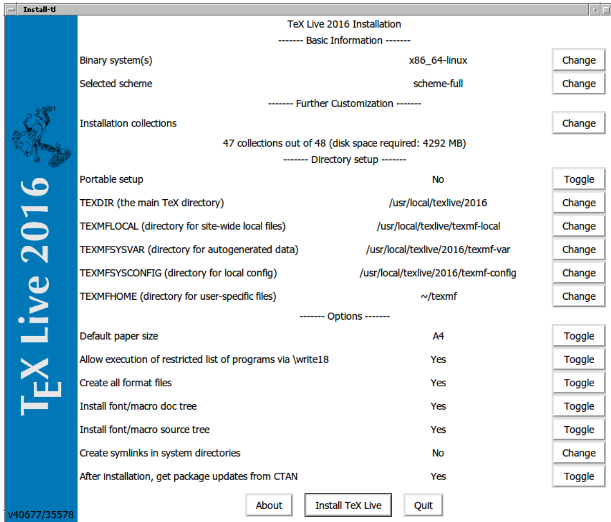
Рис. 3: Главное меню программы установки в экспертном графическом режиме (GNU/Linux)
