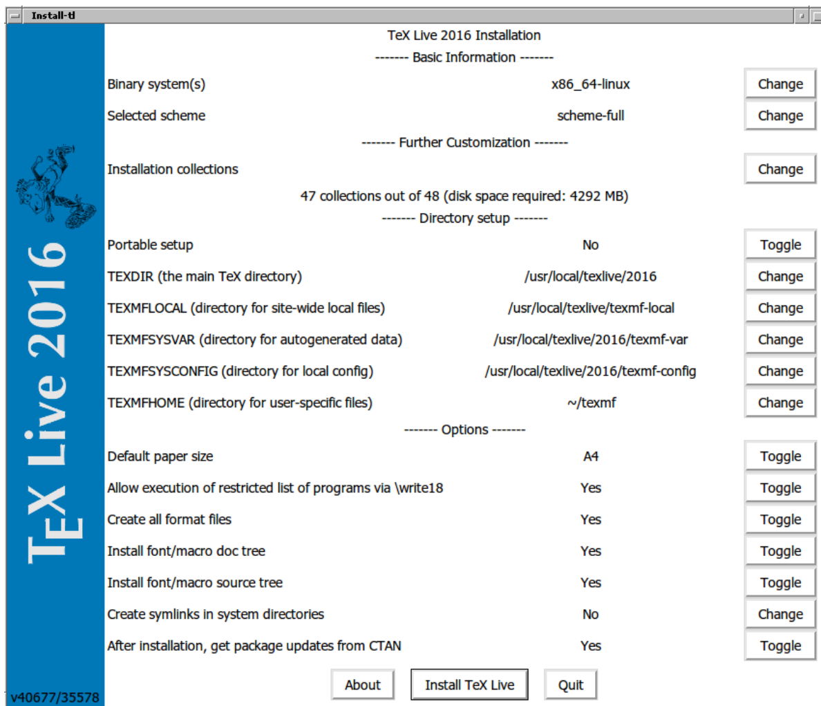
图 3: 专家模式 GUI 安装程序界面 (GNU/Linux)
