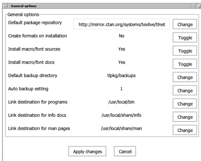
图 10: GUI 模式的 tlmgr: 通用选项
